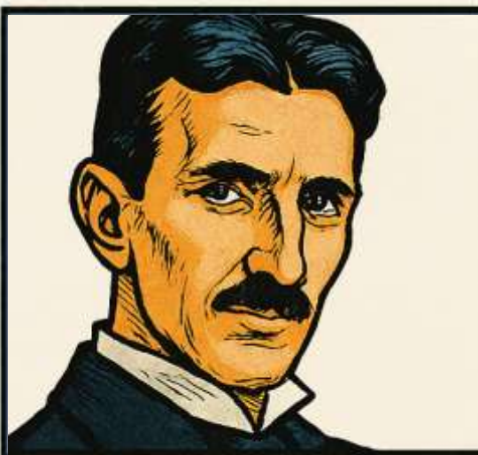
STŘÍDAVÝ PROUD
