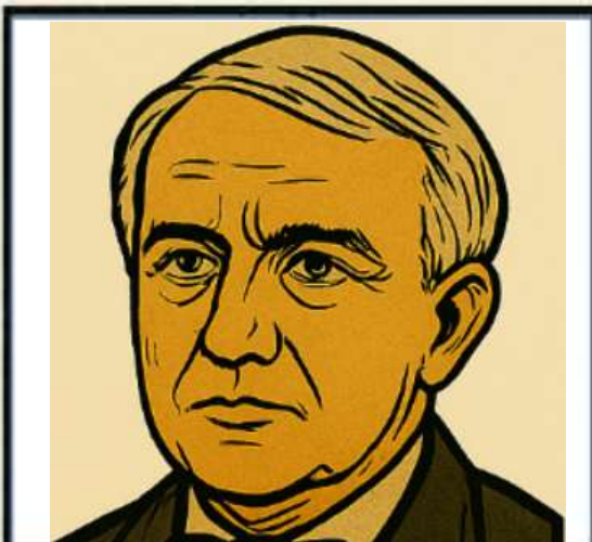
VYNÁLEZ ŽÁROVKY
