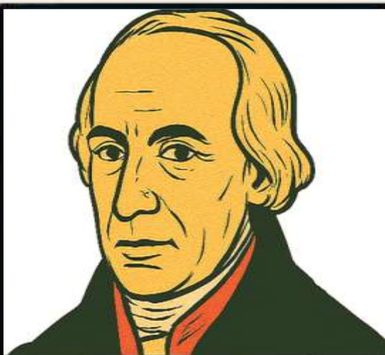
EL. NAPĚTÍ, EL. ČLÁNEK
