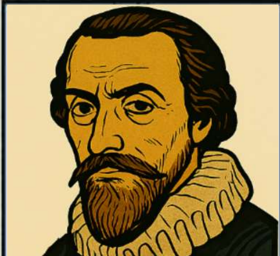
KEPLEROVY ZÁKONY PLANET
