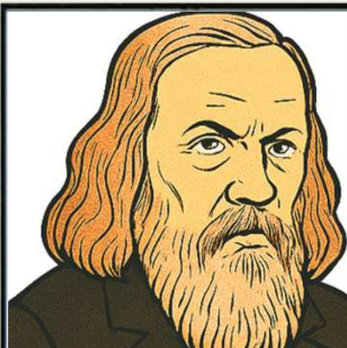
CHEMICKÁ TABULKA PRVKŮ
