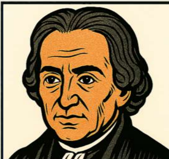
ŽABÍ STEHÝNKA A EL. PROUD
