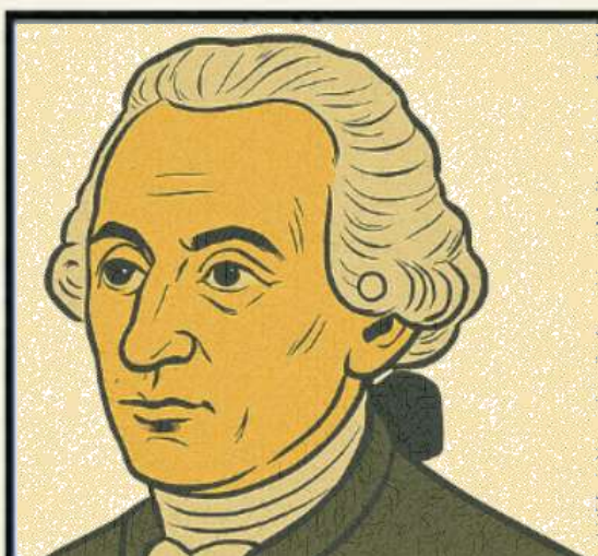
ZÁKON ZACHOVÁNÍ HMOTNOSTI
