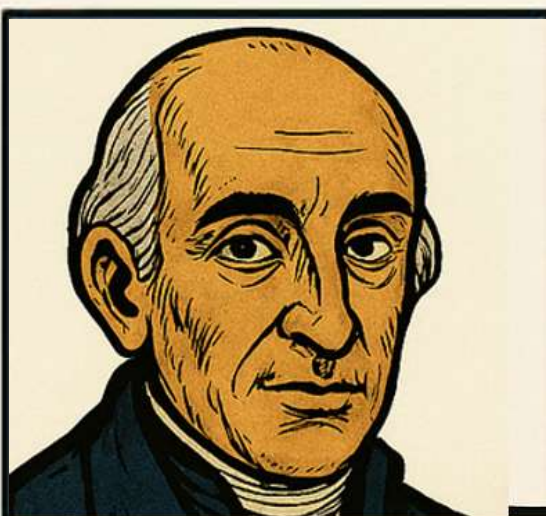
ELEKTRICKÝ NÁBOJ
