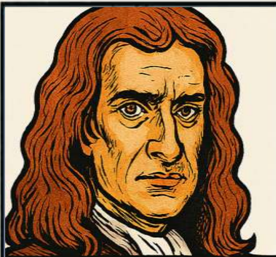
GRAVITACE, POHYBOVÉ ZÁKONY
