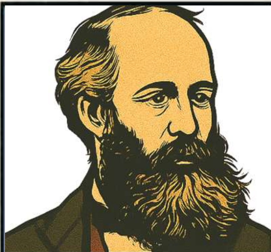
ROVNICE EM VLNĚNÍ
